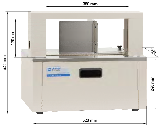
ATS-MS 380 / 35 kg
